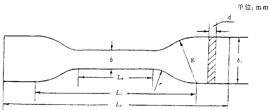
L_2 -总长 120; L_1 -夹具间初始距离 86\pm 5 ; L_0 -标线间距离 40\pm 0.5 ; d -厚度; R -大半径 25\pm 2 ; r -小半径 14\pm 1 ; b -平行部分宽度 10\pm 0.5 ; b_1 -端部宽度 25\pm 0.5
