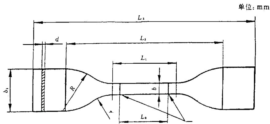
L_3 -总长 115; L_2 -夹具间初始距离 80 \pm 5 ; L_1 -平行部分长度 33 \pm 2 ; L_0 -标线间距离 25 \pm 0.25 R -大半径 25 \pm 2 ; r -小半径 14 \pm 1 ; b -平行部分宽度 6 \pm 0.4 ; b_1 -端部宽度 25 \pm 1 ; d -厚度
