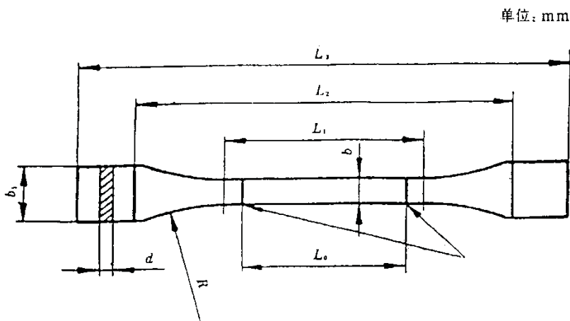
L_3 -总长 150; L_2 -夹具间初始距离 115 \pm 5 ; L_1 -平行部分长度 60 \pm 0.5 ; d -厚度 L_0 -标线间距离 50 \pm 0.55 ; R -半径 60; b -平行部分宽度 10 \pm 0.5 ; b_1 -端部宽度 20 \pm 0.5
