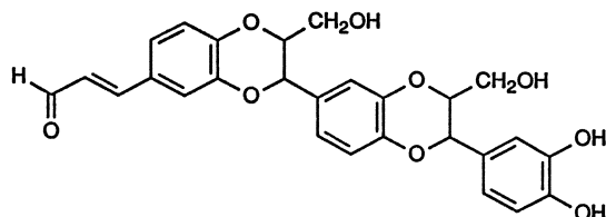
Americanin B (97-26)
