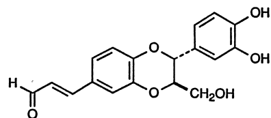
Americanin A (97-25)
