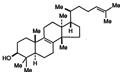
Tirucallol (97-19)
