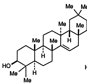
Taraxerol (97-23)
