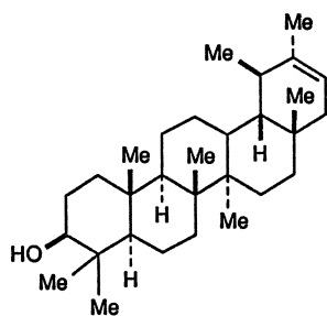
ψ-Taraxasterol (97-22)
