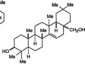
Myricadiol (97-24)
