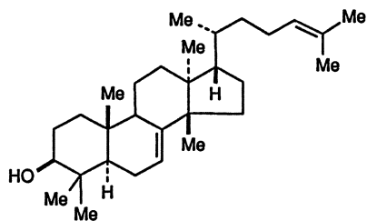
Butyrospermol (97-18)
