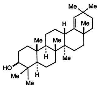
Germanicol (97-20)
